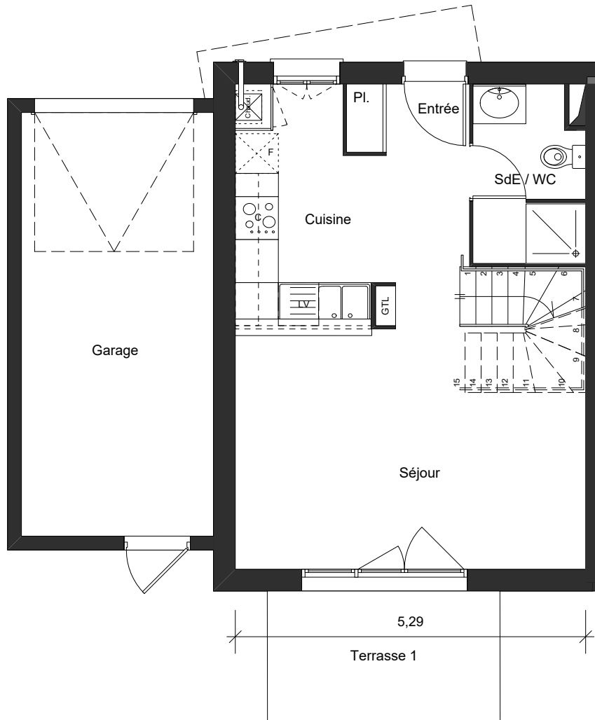
REZ-DE-JARDIN
