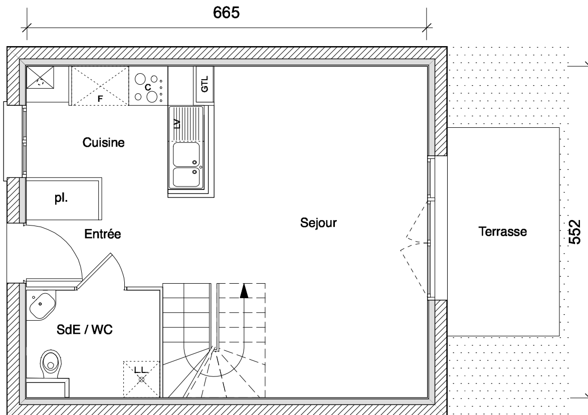
REZ-DE-JARDIN
