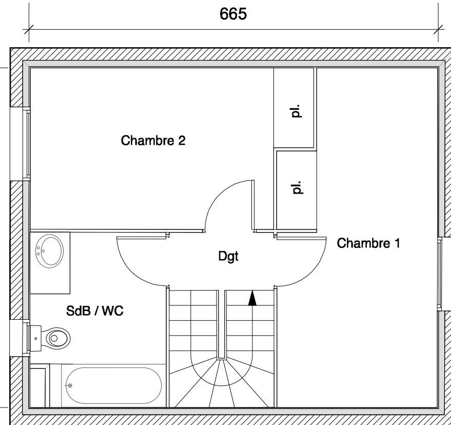
ETAGE
