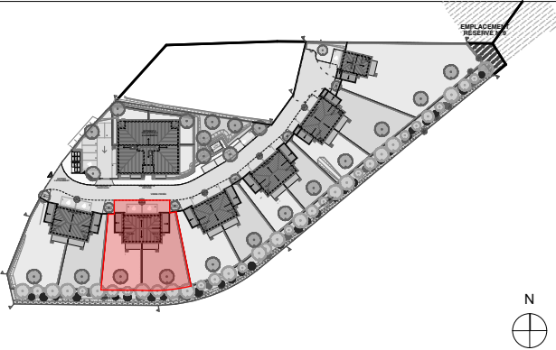
PLAN MASSE BATIMENT B2 - 2 MAISONS Type T4
