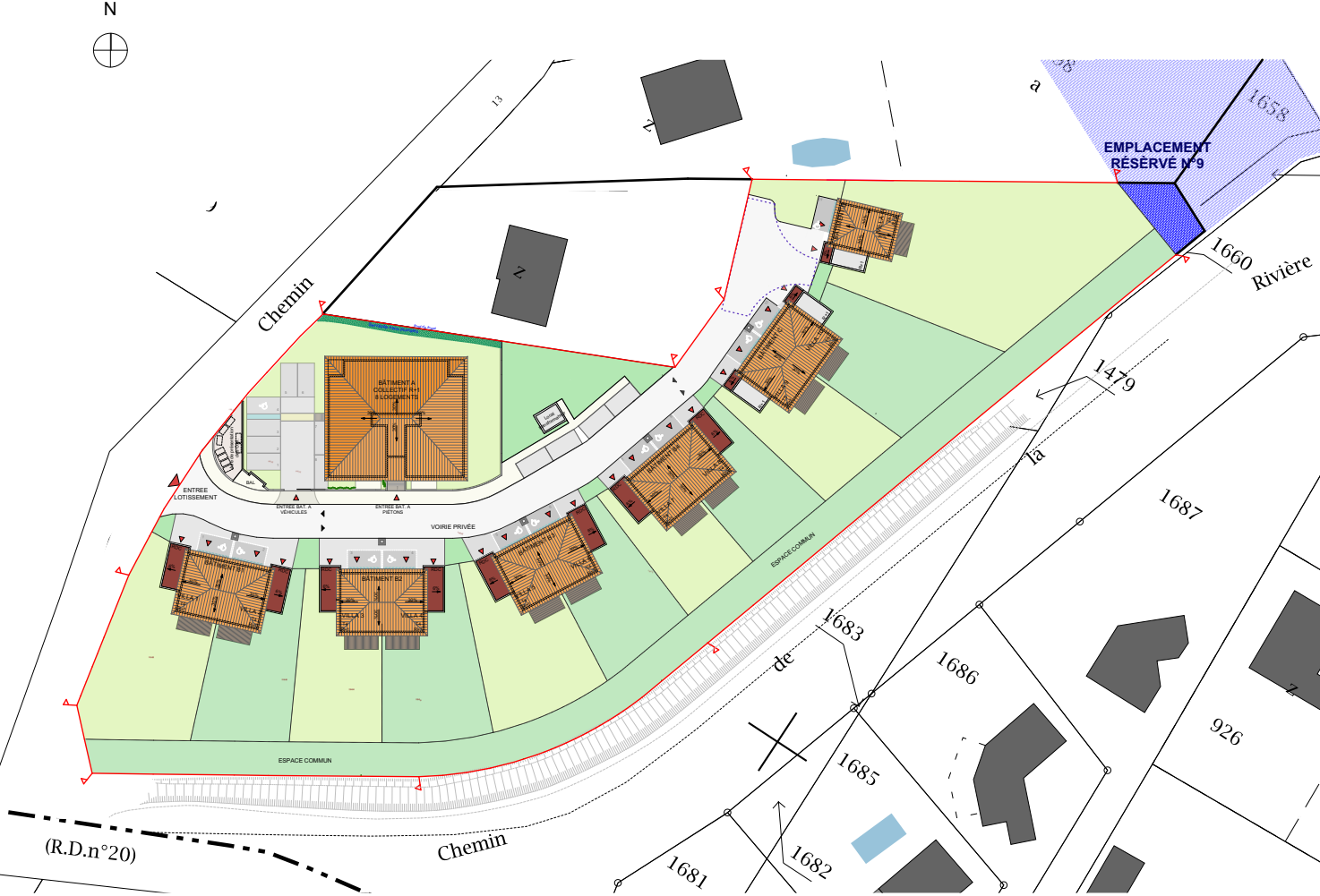
PLAN DE MASSE GENERAL
